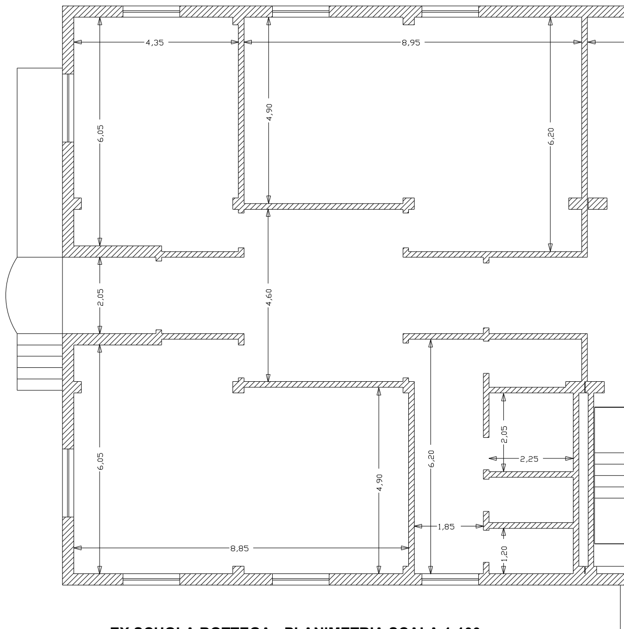
EX SCUOLA BOTTEGA - PLANIMETRIA SCALA 1:100
